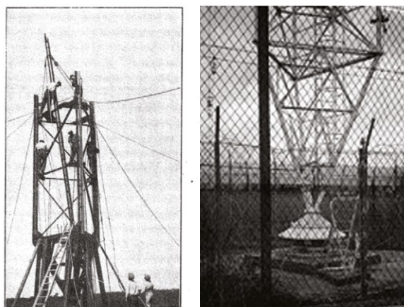
La base du pylône posée sur 3 porcelaines
